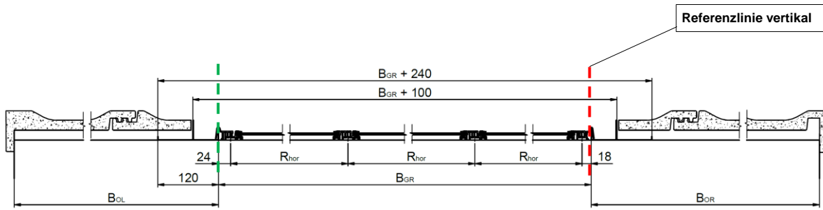
Abbildung: Horizontalschnitt Solrif
